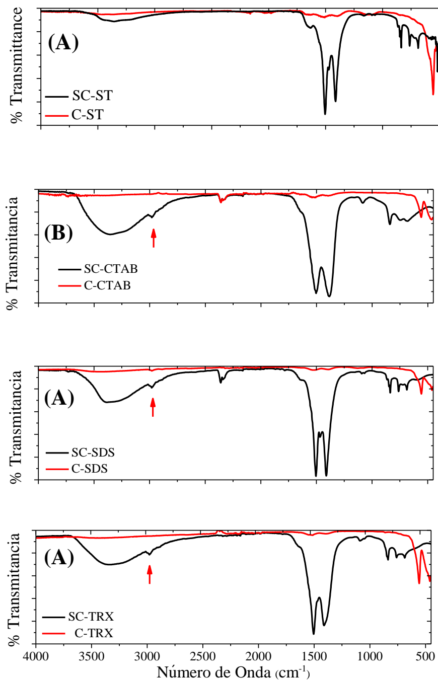
Figura 6. 3. Espectros FTIR-ATR de los precursores sin calcinar (Negro) y los óxidos de Y_2O_3:Eu^{3+} ya estabilizados térmicamente a 900^\circ C (Rojo).
