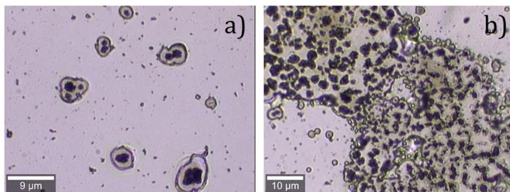
Figura 4.16.- Micrografías ópticas del área activa después de aplicar ciclos WRER. a) Burbujas reventadas y b) daño por exceso de calor al área activa.
