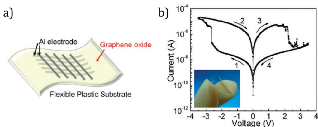
Figura 2.18.- a) Ilustración esquemática de un dispositivo de crossbar flexible basado en GO. b) Curva I-V típica de un dispositivo Al/GO/Al/PES trazada en una escala semilogarítmica. Las flechas indican la dirección de barrido de voltaje. El recuadro de la izquierda es una imagen real de un dispositivo [47].
